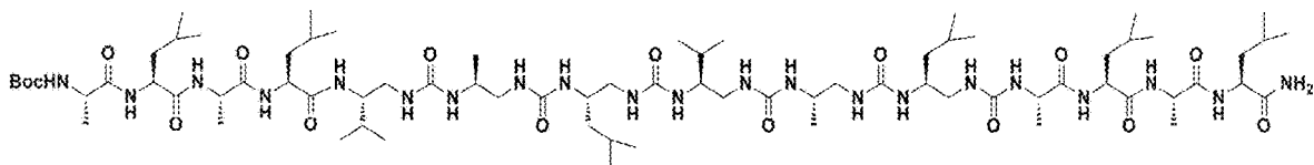
oligomer 13
