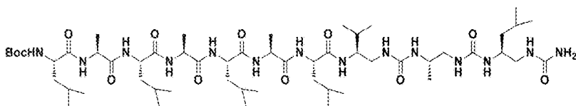
oligomer 12
