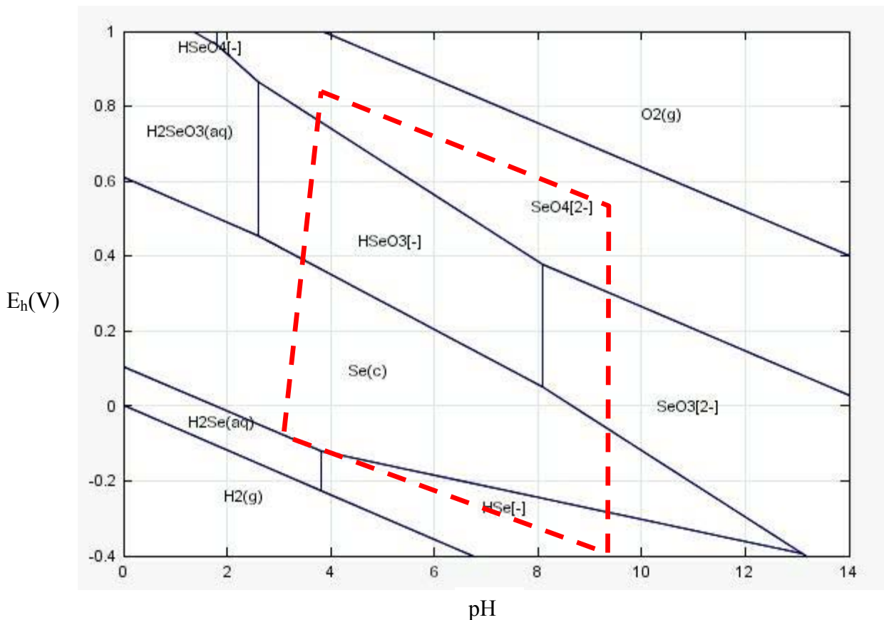
Figure 1.1 Diagramme Eh-pH du sélénium obtenu avec le logiciel JChess et la base de donnée thermodynamique décrite au chapitre 2.2.3. [Se]=50 nM. La zone en rouge représente la zone d'oxydo-réduction susceptible d'être rencontrée dans l'environnement.
