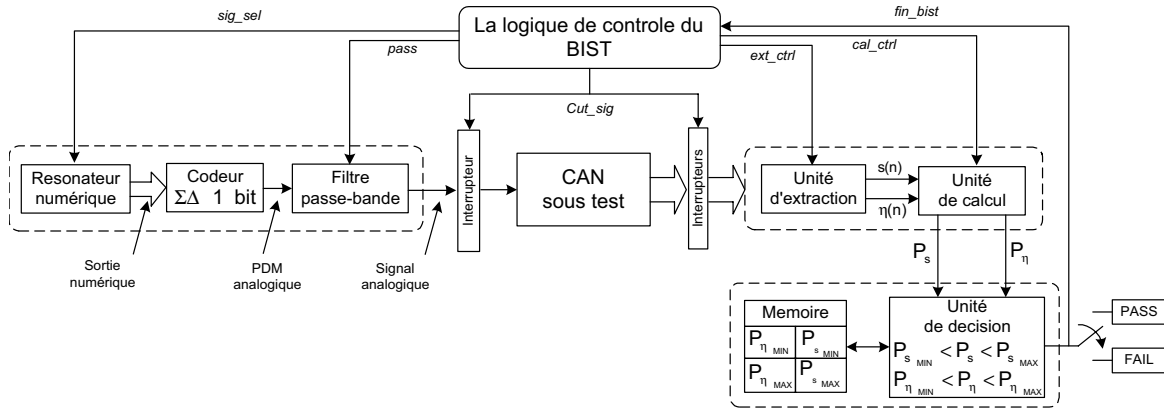
Figure 1.13 : Le schéma Bloc du BIST.
