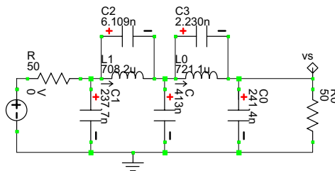
Figure B.13: filtre passe-bas elliptique du 5 e ordre.
