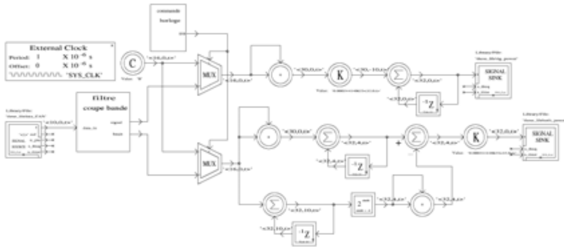
Figure IV. 26 : Calcul des puissances du fondamental et du bruit.
