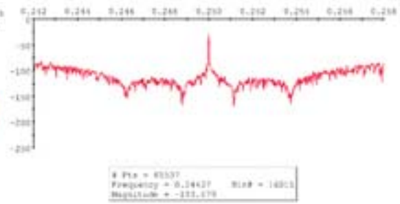
Figure IV. 10 : Allure du spectre dans la bande utile sous SPW.
