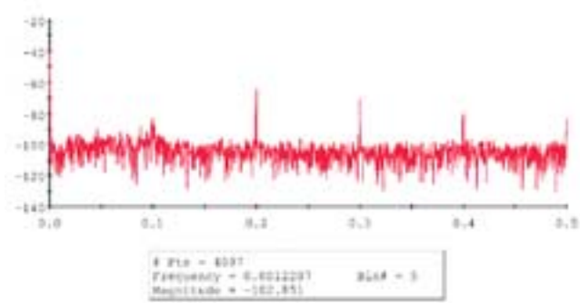
Figure IV. 25 : Spectre du signal à la sortie coupe bande du filtre.
