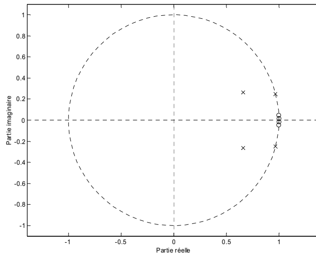
Figure II. 31 : Lieu de pôles de la NTF après quantification.
