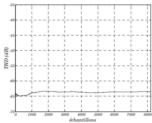
Figure III. 34 : Courbe d'évolution temporelle de la THD.
