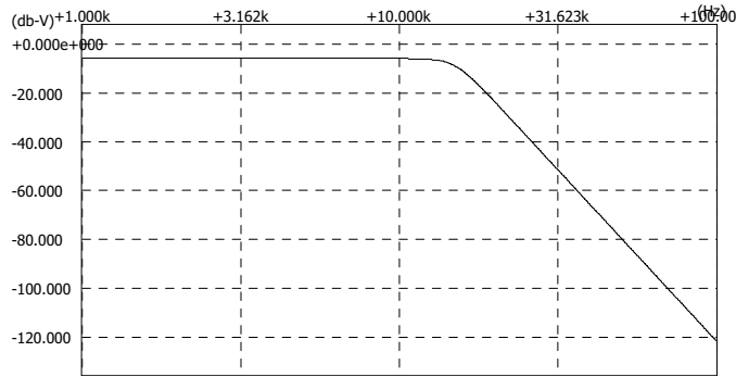
Figure B.8 : courbe de réponse du filtre de Butterworth.
