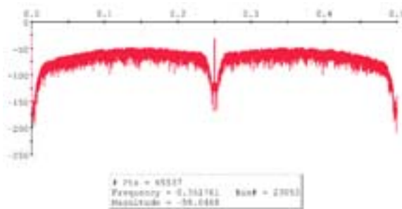
Figure IV. 9 : Allure du Spectre du signal à la sortie du modulateur \Sigma\Delta passe bande sous SPW.
