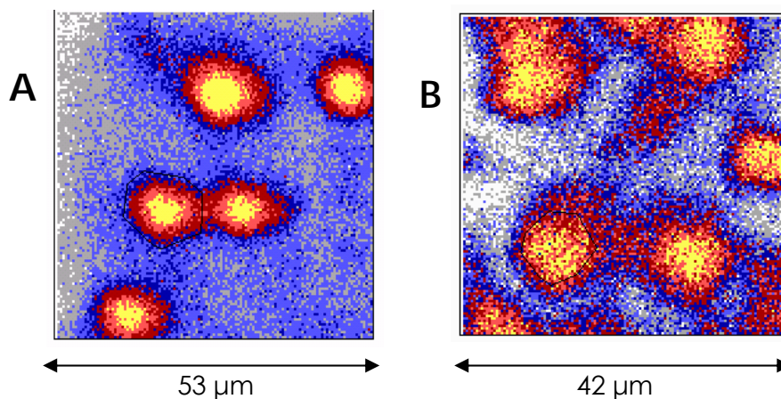
Figure 18 : Microanalyse en microscopie ionique (RBS) de cellules HaCaT/[H2B-GFP]Tg . Les cellules ont été cryofixées après 4h (A) et 24h (B) de culture sur membrane de polycarbonate/Cell-Tak. Représentation de la distribution en concentration du carbone. L'échelle de couleur est définie de manière à ce que la concentration augmente du blanc au jaune
