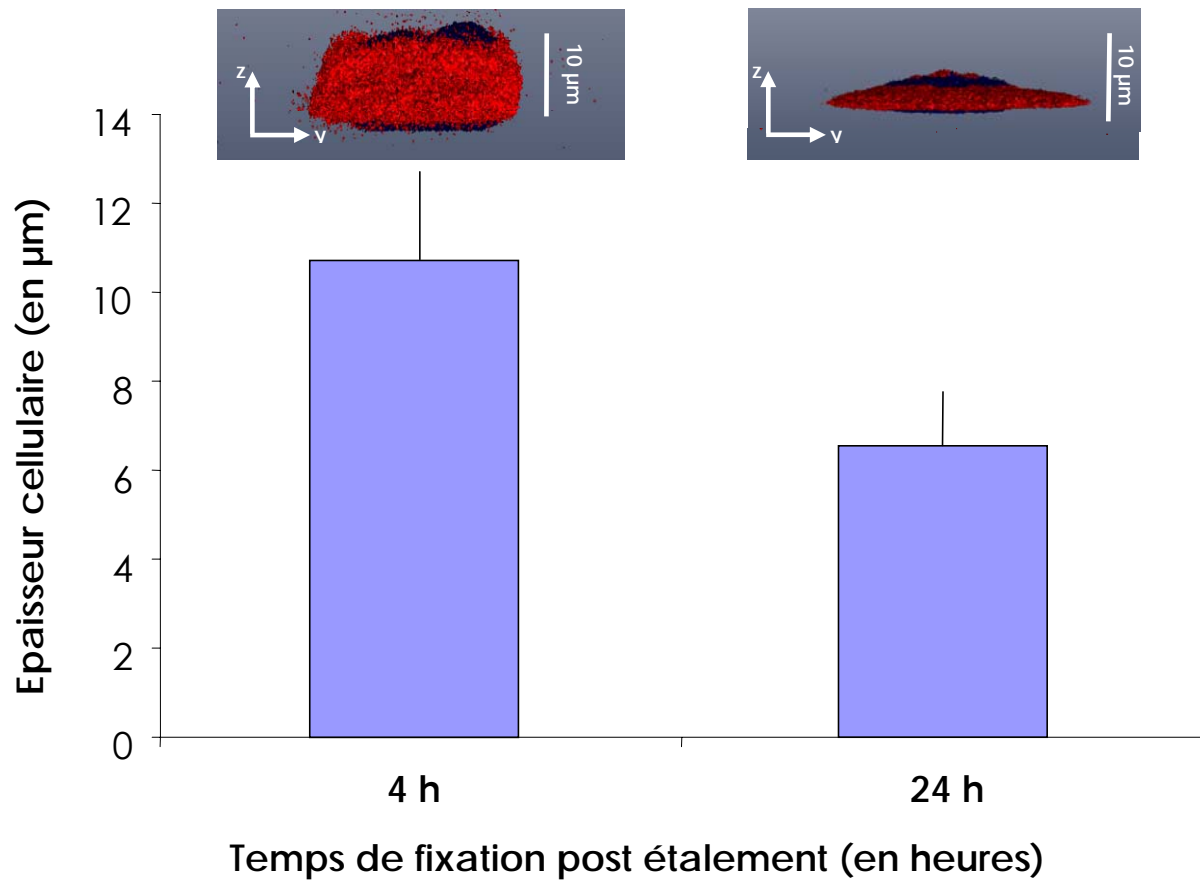
Figure 17 : Epaisseur cellulaire moyenne . Mesure de l'épaisseur des cellules HaCaT/[H2B-GFP]Tg étalées sur membrane de polypropylène/Cell-Tak sur des images de microscopie confocale. La mesure de l'épaisseur de chaque cellule est effectuée et montre une épaisseur de 10.70 µm (+/- 1.97 µm, n=12) pour les cellules étalées 4 heures et de 6.54 µm (+/- 1.20 µm, n=46) pour les cellules étalées 24 heures.
