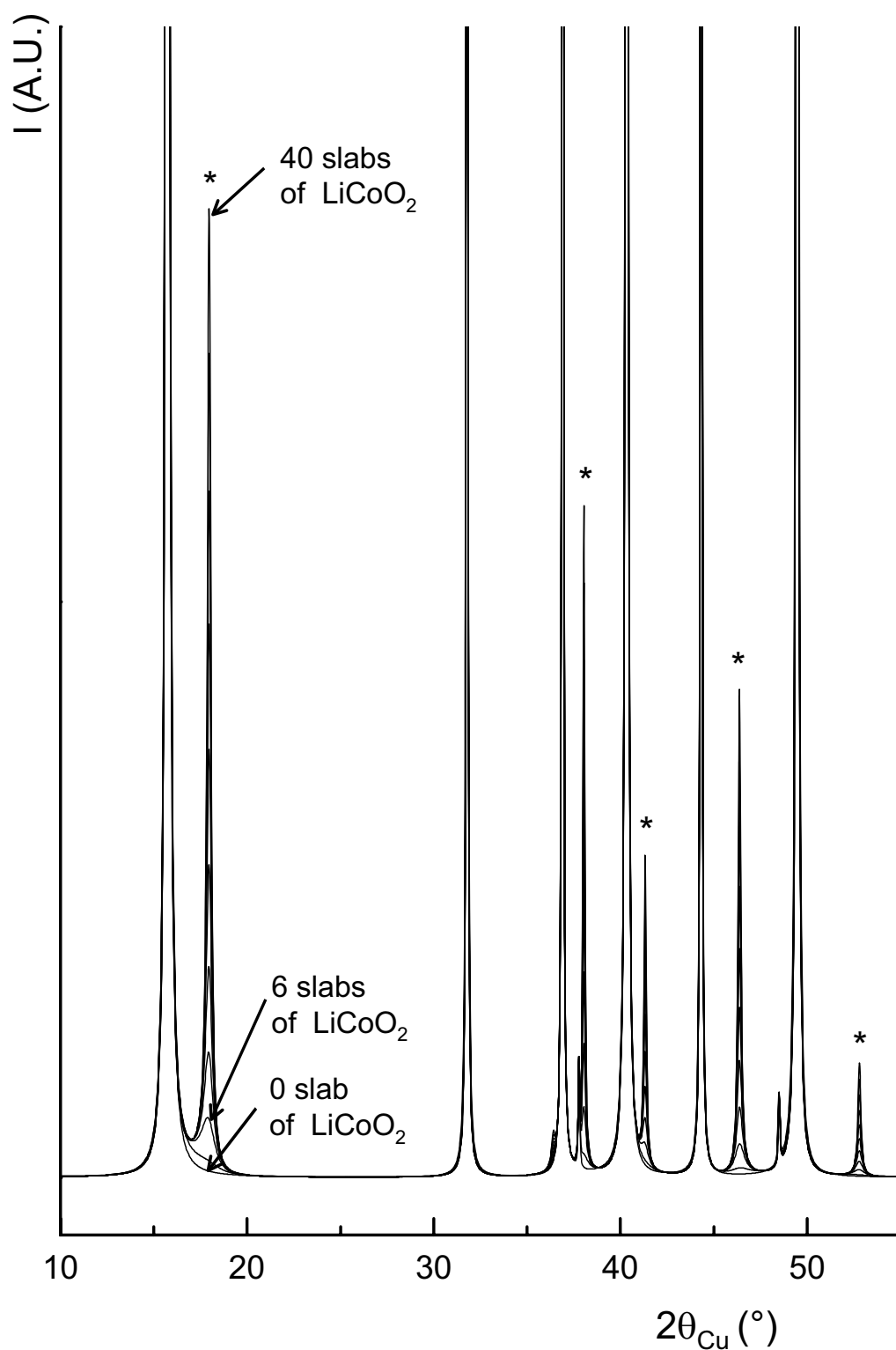
Fig. A-II 7 : Diagrammes de diffraction des rayons X calculés pour l'intercroissance P2 - O2. Les "*" indiquent la position des raies de diffraction de O2-LiCoO 2 . La taille moyenne des domaines O2 varie entre 0 et 40 feuillets.
