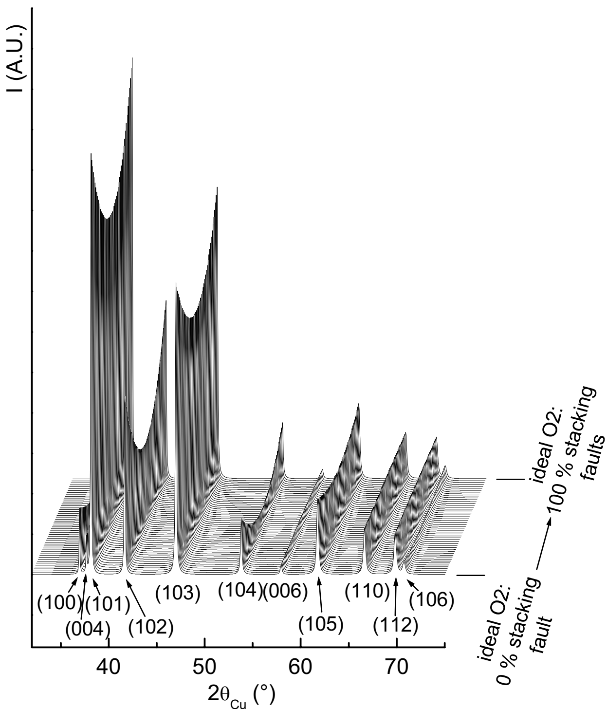
Fig. A-I 5 : Diagrammes de diffraction des rayons X calculés pour O 2 -LiCoO 2 avec des fautes d'empilement, en considérant que les centres de nucléation sont associés à un seul type de feuillets (AB ou BA). Les vecteurs de glissement sont (1/3, 2/3, 0) ou (2/3, 1/3, 0) . La raie de diffraction (002) qui n'est pas affectée par les défauts n'est pas représentée sur la figure.
