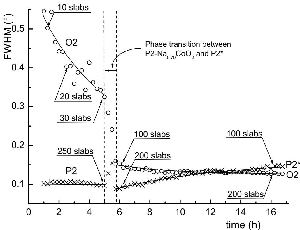
Fig. A-II 4 : Evolution des FWHM des raies de diffraction (002) associées aux phases \text{P2-Na}_{0.70}\text{CoO}_2 (x), \text{P2}^*\text{-Na}_{0.50}\text{CoO}_2 (o) et \text{O2-LiCoO}_2 (°), pendant la réaction d'échange ionique. Les longueurs de cohérence calculées avec la formule de Scherrer à partir des valeurs de FWHM expérimentales sont aussi indiquées.
