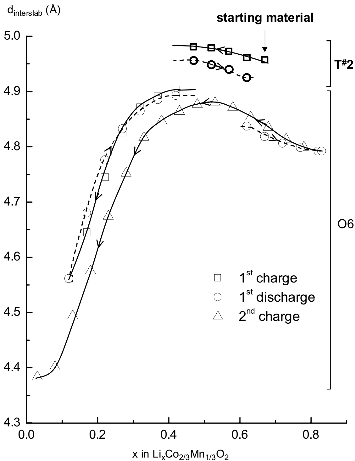
Fig. B-II 7 : Evolution de la distance interfeuillet (paramètre c / nombre de feuillets nécessaires pour décrire la maille) en fonction de la concentration en lithium dans Li x Co 2/3 Mn 1/3 O 2 . Le domaine T # 2 est représenté en traits gras.
