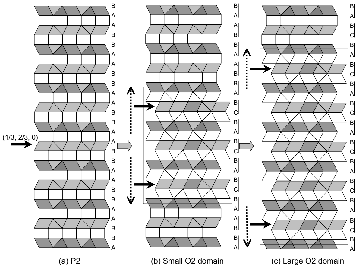
Fig. A-I 2 : Un exemple de croissance de domaines O 2 dans un cristal P 2 , à partir de centres de nucléation de type BA. Le même vecteur de glissement (1/3, 2/3, 0) (flèche noire) est conservé pour le domaine entier de croissance.
