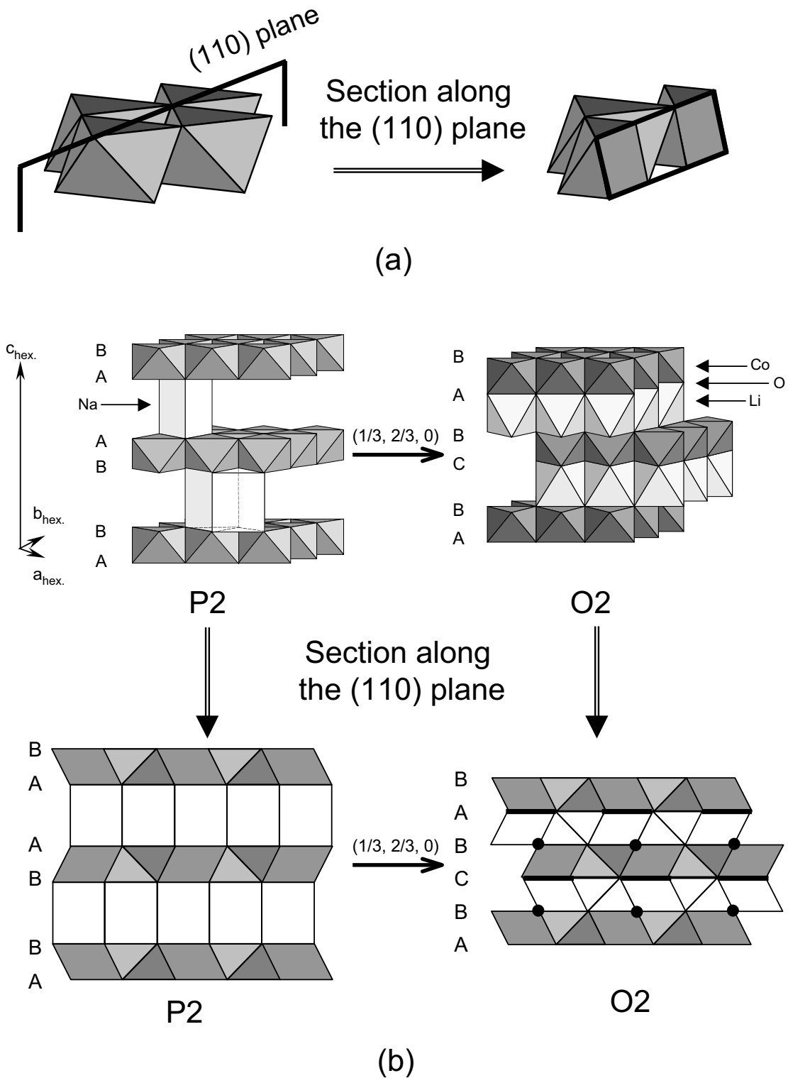
Fig. A 1 : (a) Section d'un feuillet MO_2 dans le plan (110). (b) Glissement de feuillets mis en jeu lors de la transition P2 \rightarrow O2 : représentation en perspective et en coupe selon la section dans le plan (110). Une face commune apparaît comme un segment partagé entre deux parallélogrammes (—) alors qu'une arête commune apparaît comme un point (•) dans la section.
