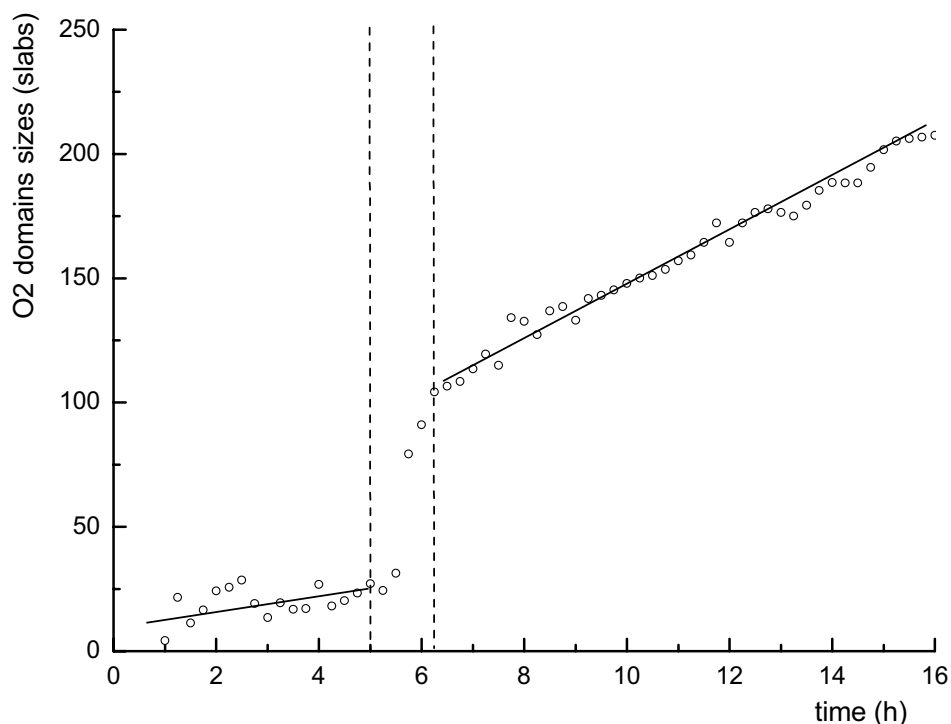
Fig. A-II 5 : Evolution de la taille moyenne des domaines O2 (en nombre de feuillets) pendant l'échange ionique.
