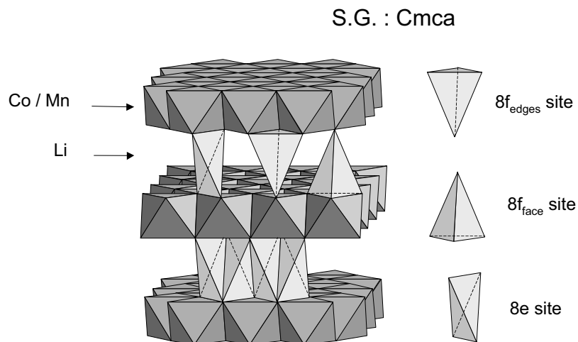
Fig. B-I 4 : Empilement oxygéné T#2 de la phase \text{Li}_{2/3}\text{Co}_{2/3}\text{Mn}_{1/3}\text{O}_2 . Les différents sites tétraédriques accessibles pour les ions lithium sont aussi représentés.
