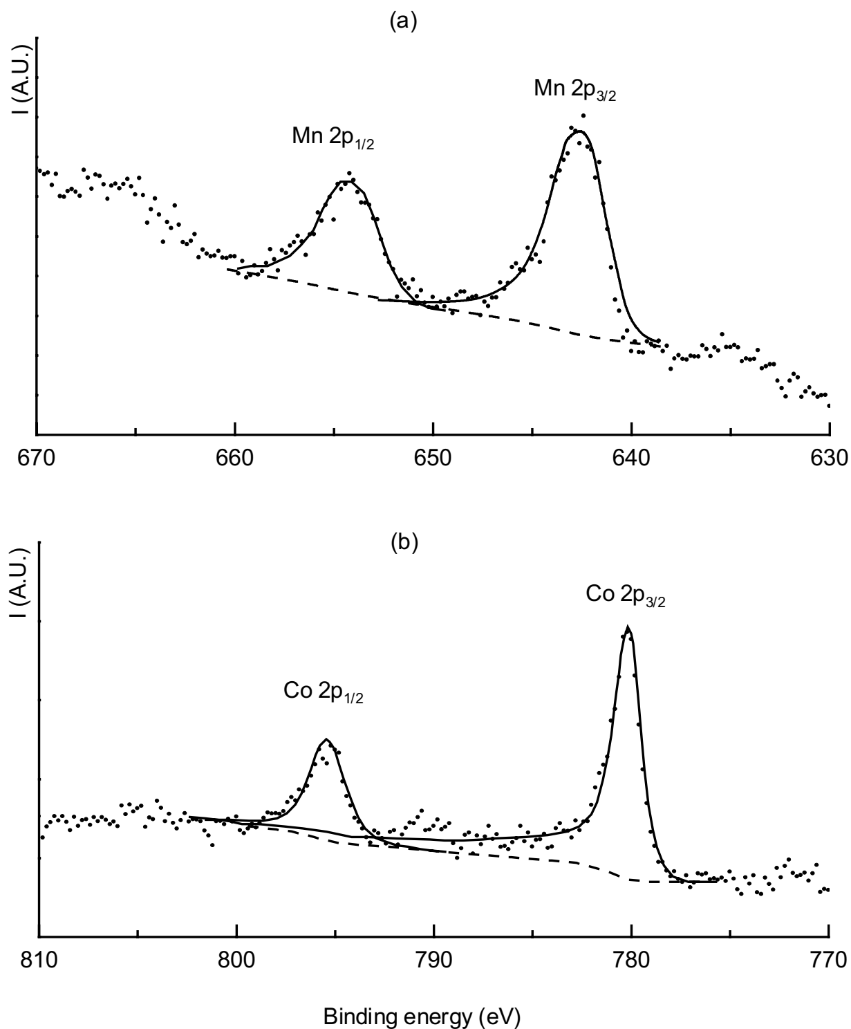
Fig. B-I 6 : Comparaison des spectres XPS Mn 2p (a) et Co 2p (b) calculés (-) avec les données expérimentales (•) obtenues pour \text{T}^{\#2}\text{-Li}_{2/3}\text{Co}_{2/3}\text{Mn}_{1/3}\text{O}_2 . La ligne pointillée représente le fond continu.
