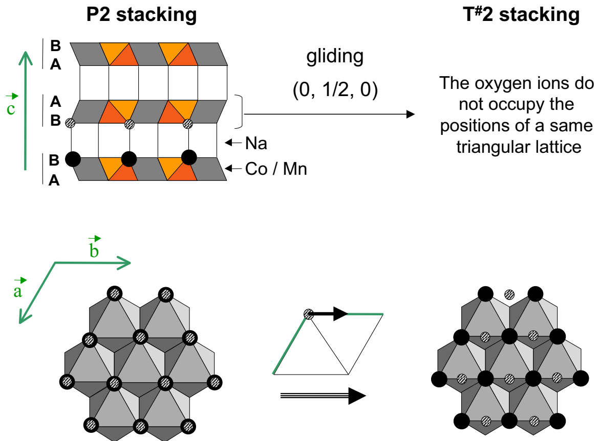
Fig. B-I 3 : Glissement de feuillets mis en jeu lors de la transition P2 \rightarrow T#2 qui a lieu pendant le processus d'échange ionique. Représentation de la section dans le plan (110) et en vue de dessus à partir d'un espace interfeuillelet. Les deux couches d'oxygène d'un espace interfeuillelet sont mises en valeur : les ions oxygène de la couche inférieure sont représentés par des disques noirs et ceux de la couche supérieure par des disques hachurés.
