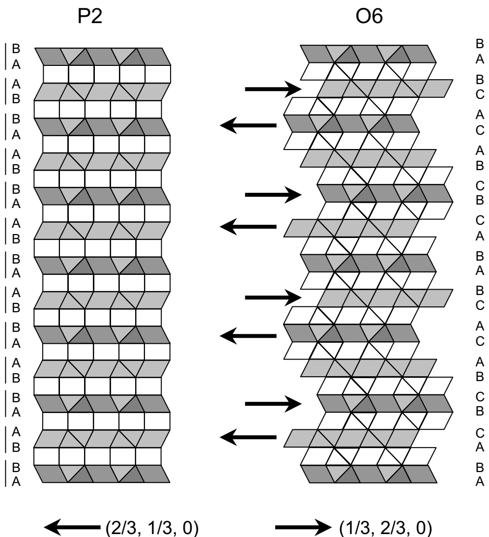
Fig. A-I 9 : Transition P2 \rightarrow O6 selon la section dans le plan (110). Les feuillets plus clairs sont de type BA, alors que les plus foncés sont de type AB. Les centres de nucléation sont associés aux deux types de feuillets (AB ou BA), les vecteurs de translation (flèches noires) sont (1/3, 2/3, 0) ou (2/3, 1/3, 0) . Pour faciliter la lecture de cette figure, les prismes de sodium sont dessinés avec la même hauteur que les octaèdres de lithium.
