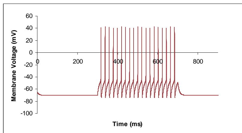
Figure 2.5. Allure des potentiels d'action sous Neuron d'un neurone excitateur
