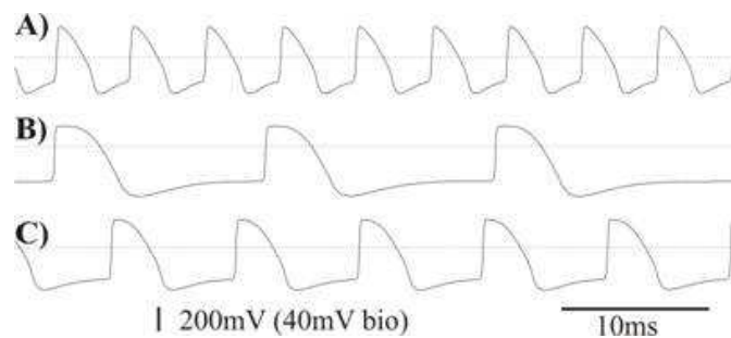
Figure 2.17. Activités de trois neurones (A, B, C) du circuit Galway
