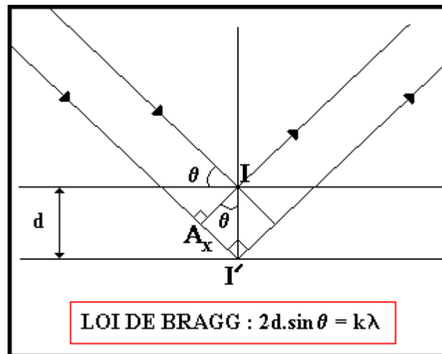
Figure 14 : Loi de BRAGG
