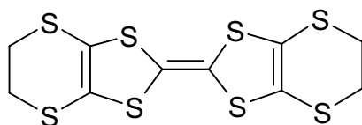
Fig. 3. Structure du donneur organique BEDT-TTF.
