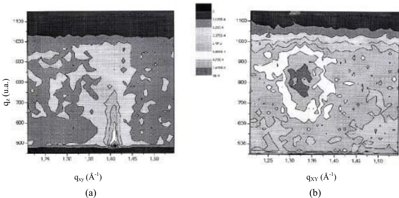
Fig. 1.16. Contour d'intensité en fonction des vecteurs (a) dans et (b) hors-plan de DODA sur une solution de \text{K}_3\text{Fe}(\text{CN})_6 \cdot 5 \cdot 10^{-6} \text{ M} à 22 \text{ mN}\cdot\text{m}^{-1} .
