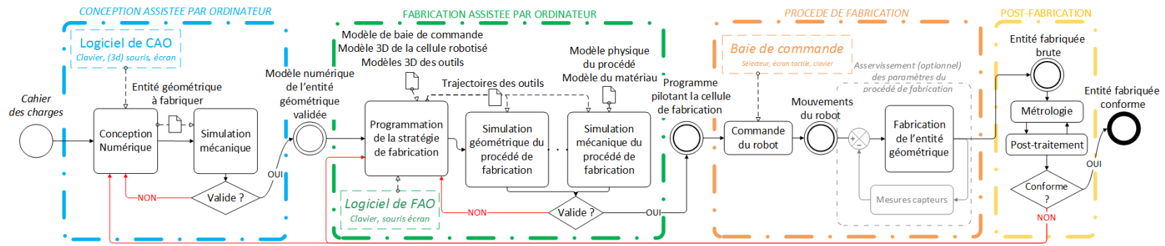
Figure 1: Le processus et le vocabulaire de la Chaîne Numérique, schématisé à partir de [2, 9].
