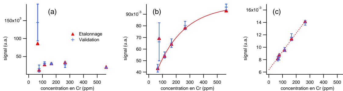
FIG. 4.13 – Courbes d'étalonnage du chrome dans le sol Bourran. Les barres d'erreur correspondent à un écart-type calculé sur les 5 spectres de validation. (a) Spectres bruts. (b) Normalisation par rapport à la raie du fer à 373.49 nm. L'ajustement exponentiel ne prend pas en compte les spectres à 76 ppm. (c) Normalisation par rapport au fer, puis par rapport à l'aire du spectre. Le coefficient de régression de la partie linéaire vaut r^2 = 0.9946 .
